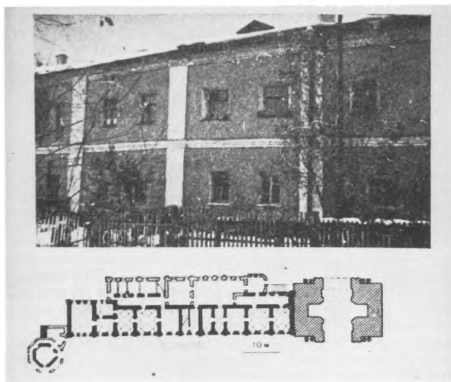
Вид и план Государевых и Патриарших палат 84
