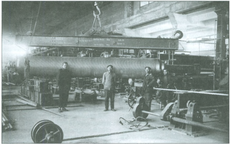
Зал буммашин. Монтаж вала Белойта. 1931 год.
