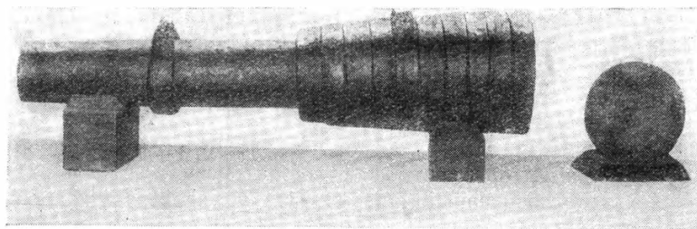
Пушка, стреляющая каменными ядрами (XV в.)
