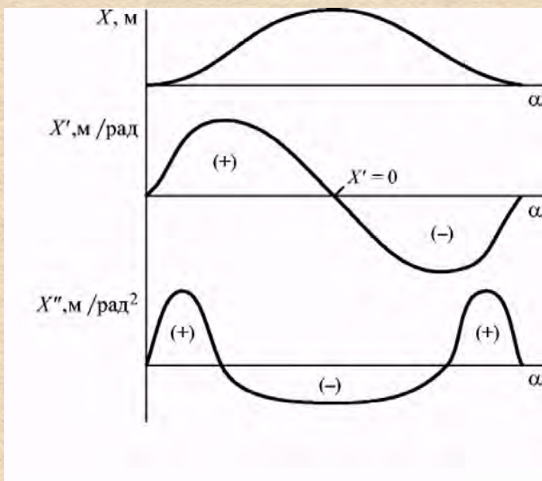
Рис.2. Характеристики закона движения толкателя
