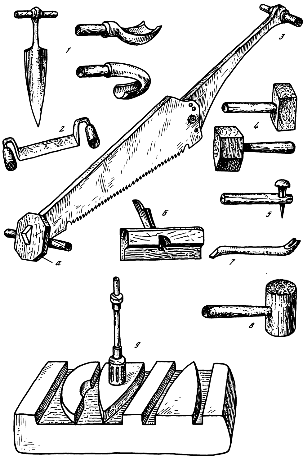
Рис. 7. Плотницкие инструменты: 1 — тесла; 2 — наструга; 3 — маховая пила; а — баклушка; 4 — кийка; 5 — бродок; 6 — голтель; 7 — выдерга; 8 — чекмарь; 9 — бало.
