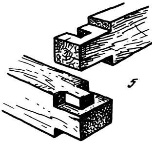
Рис. 11. Способы заделки углов в деревянных постройках: 1 — чистый угол; 2 — в охряпку; 3 — в лапу; 4 — в ласточкин хвост; 5 — потемок.
