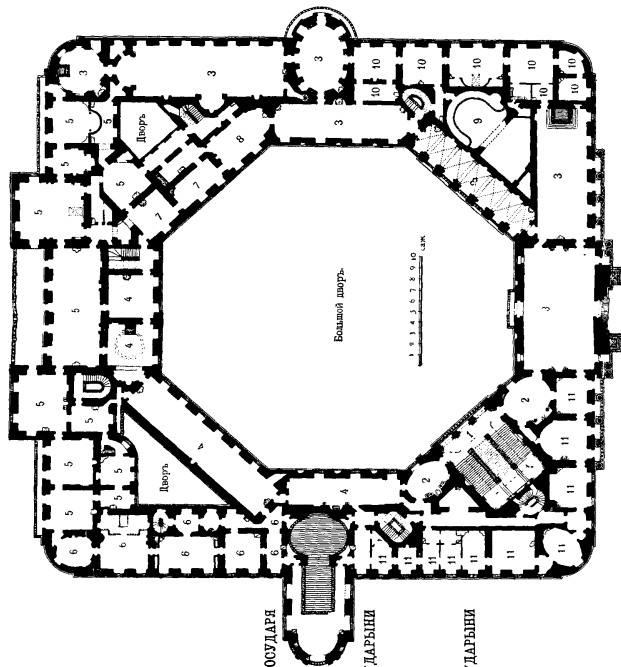
Плань бель-этажа Михайловскаго Замка.
