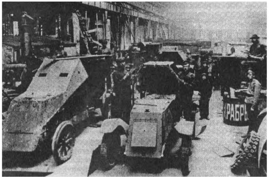
Цех бронирования автомобилей Ижорского завода (Петроград), 1915. Бронироваются автомобили: слева — «Уайт» (по системе штабс-капитана Мгбберова), справа — перебронировуется «Остин» (1-ой заготовки).
